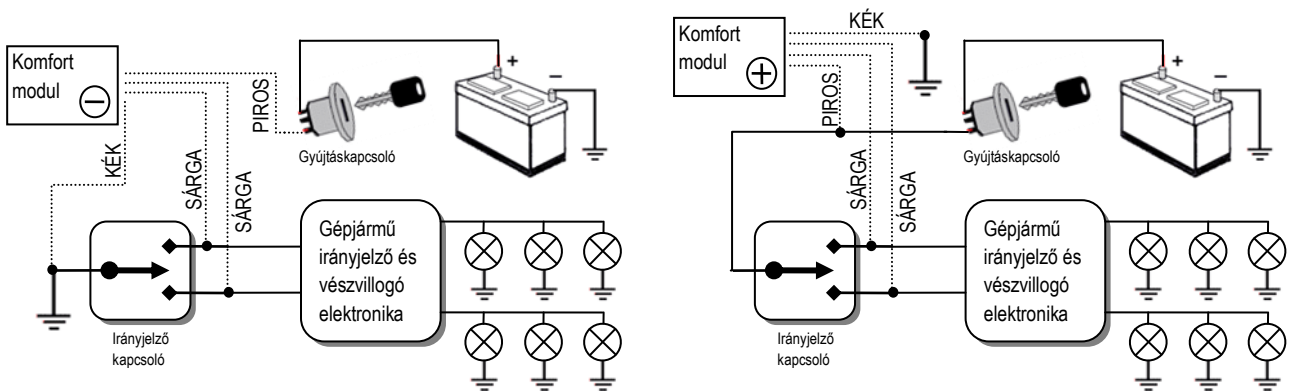
Negatív polaritású rendszer bekötése
